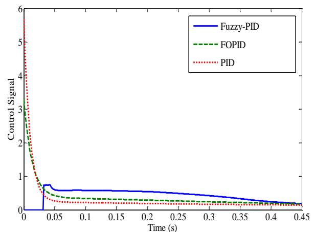
شکل ۷: سیگنال کنترلی به ازای سه کنترل کننده
