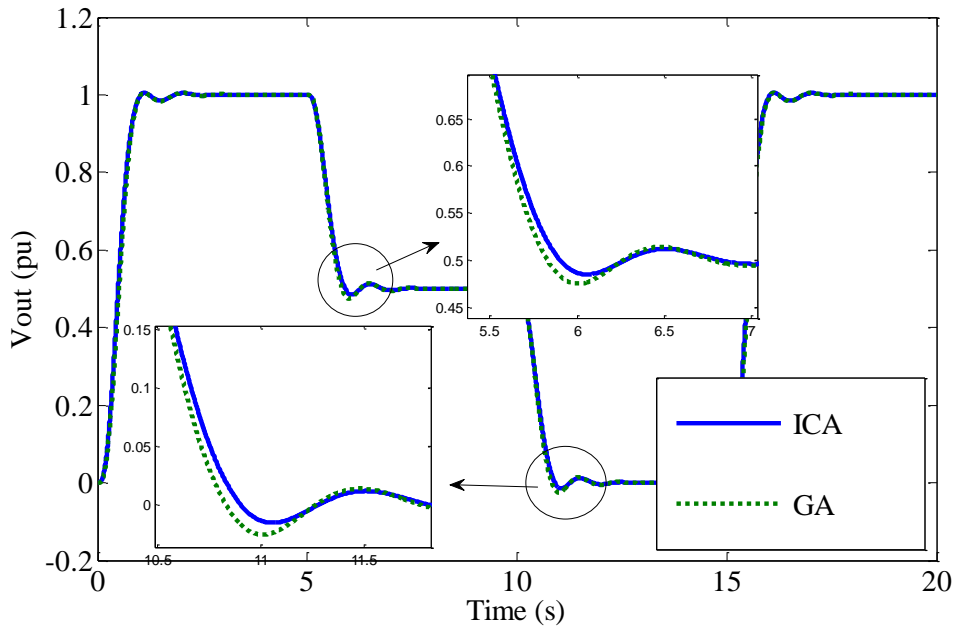
شکل ۱۸: مقایسه عملکرد کنترل کننده‌های بهینه شده با الگوریتم رقابت استعماری و الگوریتم ژنتیک در ردیابی ورودی مرجع
