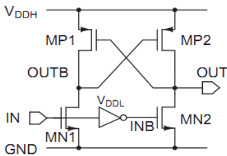
شکل ۱: تغییر دهنده سطح ولتاژ قراردادی [۱۵].
