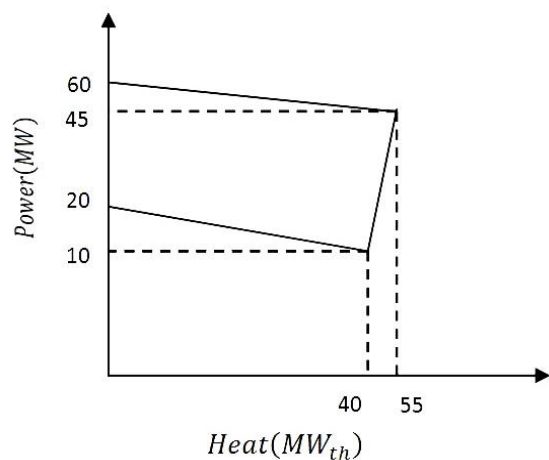
شکل ۵: ناحیه عملکرد واحد ۲
