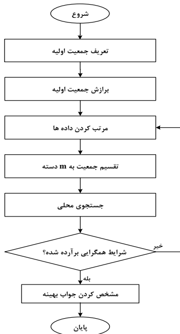
شکل ۳: فلوجارت الگوریتم جهش قورباغه
