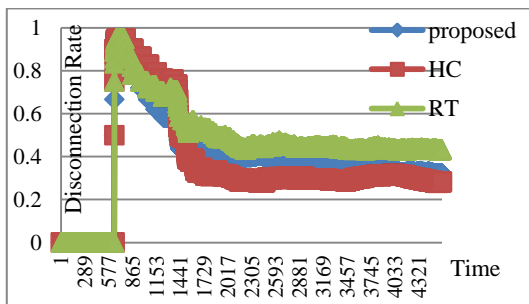
شکل ۵: نرخ قطع شدن سرویس در سناریوی ۲
