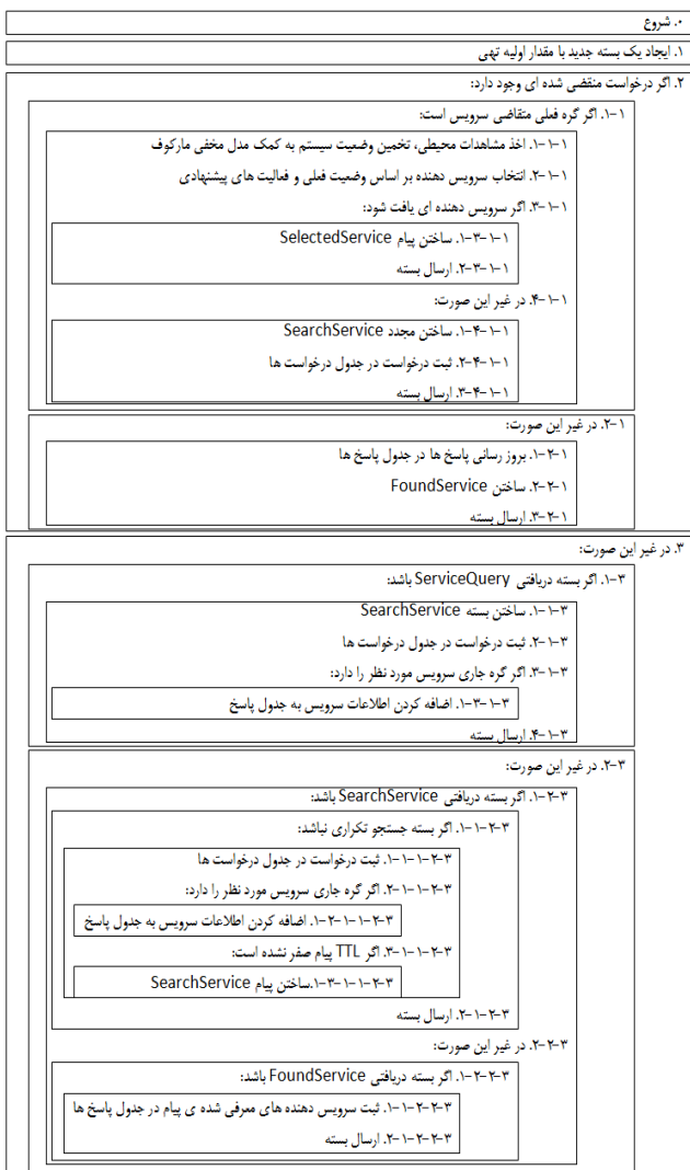
شکل ۲: الگوریتم پیشنهادی
