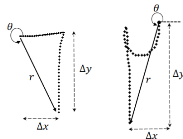
شکل ۷: نحوه استخراج ویژگی‌های سراسری.
