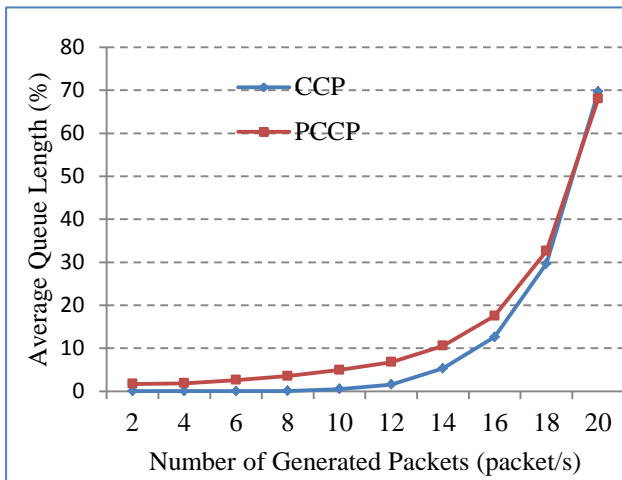
شکل ۱۵: طول صف بر اساس نرخ بسته‌های تولیدی
