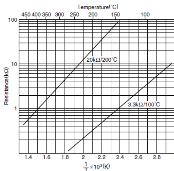
شکل ۱: منحنی تغییرات مقاومت NTC نسبت به حرارت
