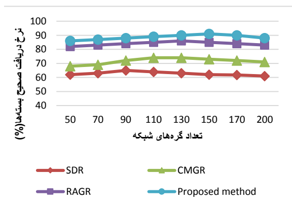
شکل ۳: مقایسه نرخ دریافت صحیح بسته روش پیشنهادی با روش‌های مورد مقایسه با ۲۰۰ خودرو.
