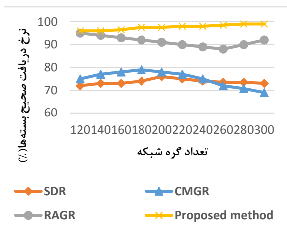
شکل ۴: مقایسه نرخ دریافت صحیح بسته روش پیشنهادی با روش‌های مورد مقایسه با ۳۰۰ خودرو.
